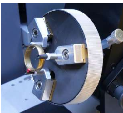
旋转辅助器
